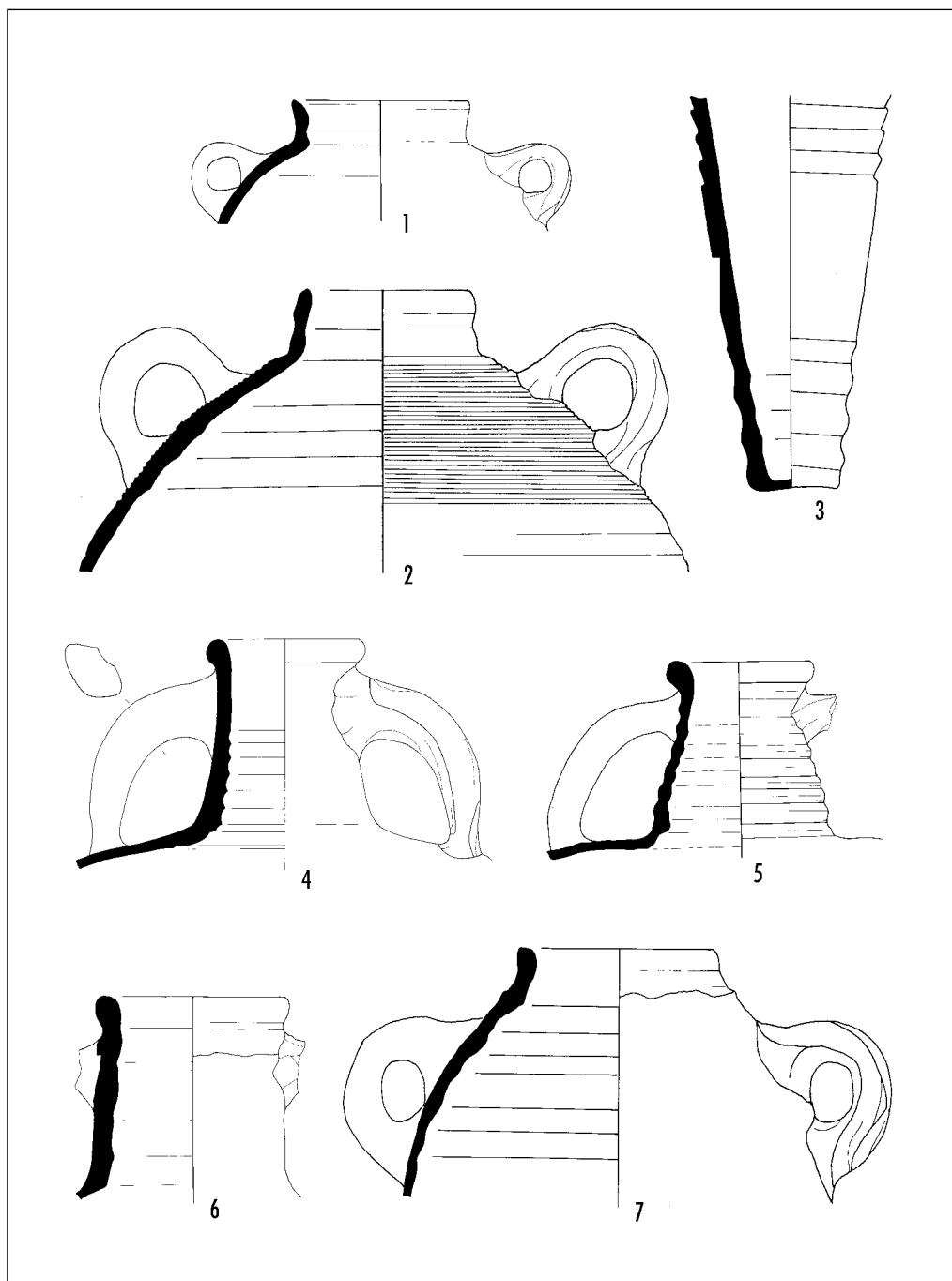
Fig. 2. Amphorae types: 2:1,2 – LRA 5/6; 2:3 – LRA 7; 2:4,5 – Kellia 167; 2:6 – LRA 1; 2:7 – LRA 4. Scale 1:4 (Drawing G. Majcherek)
